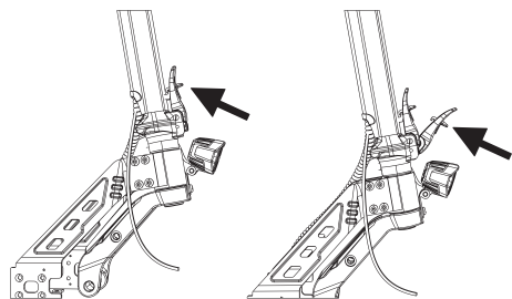
2. Öffnen Sie den Klappverschluss und klappen Sie die Vorderseite des Fahrzeugs zusammen.
