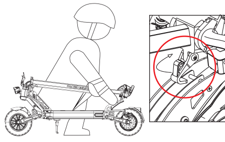
3. Klappen Sie den Fahrzeugkörper zusammen und haken Sie den Haken in die entsprechende Position ein.
